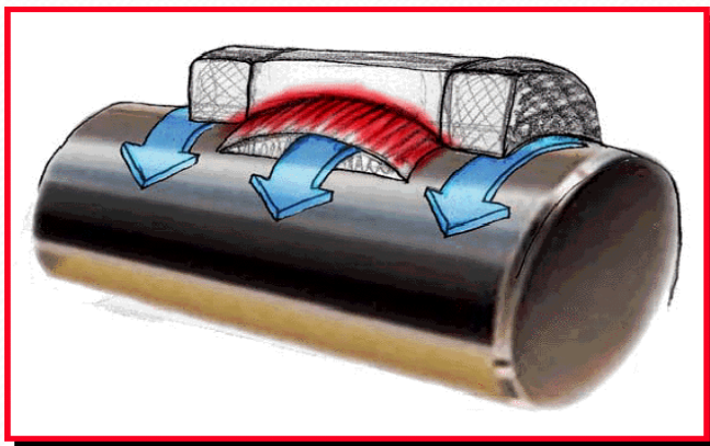
Desgaste do eixo com gaxeta Injetável
